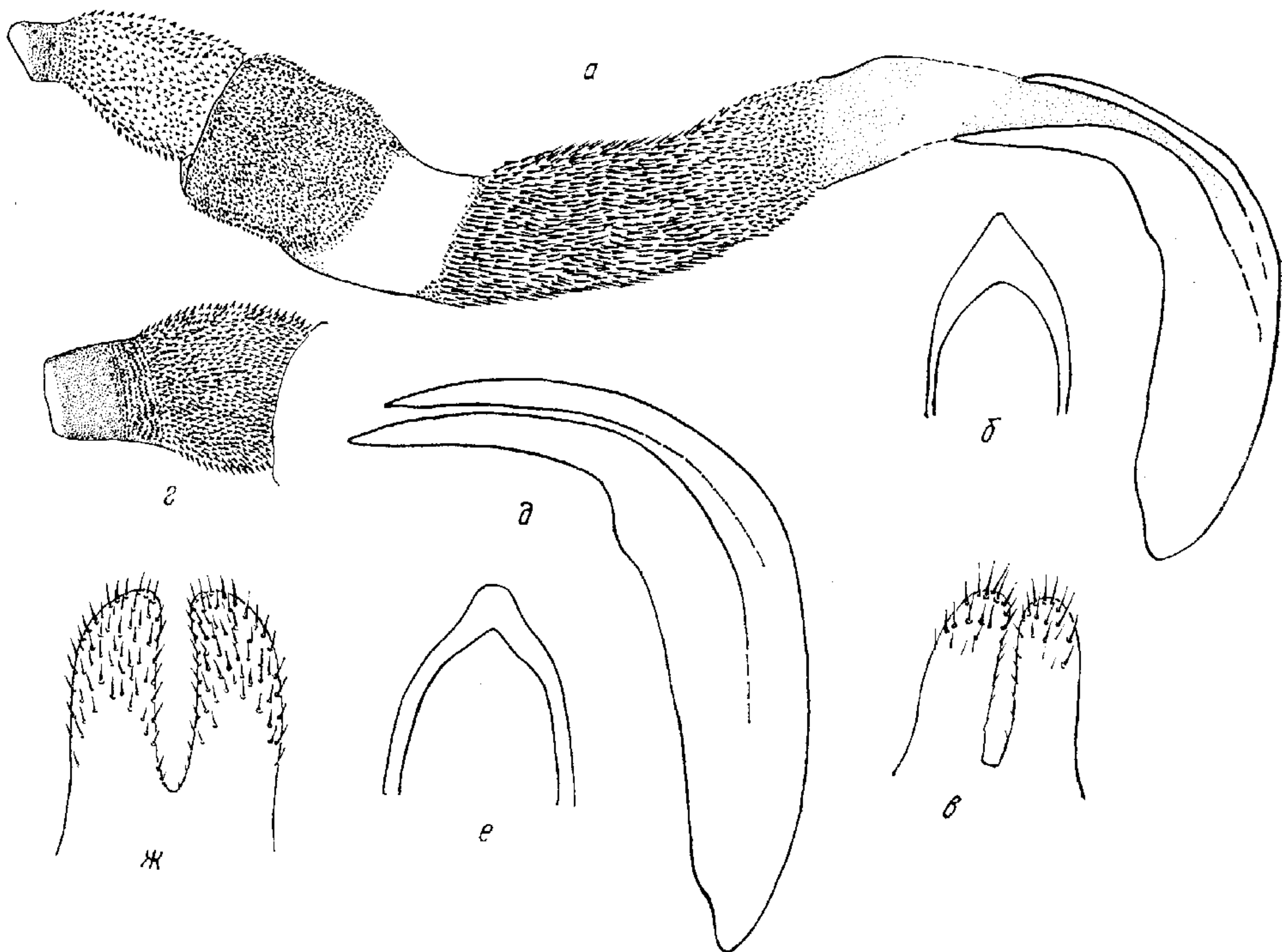
Рис. 2. Детали строения гениталий самцов Dorcadion alakoliense Danilevsky, sp. n. (а — эндофаллюс и пенис; б — вершина пениса; в — парамеры) и D. cephalotes (г — апикальный мешок эндофаллюса; д — пенис; е — вершина пениса; ж — парамеры).
