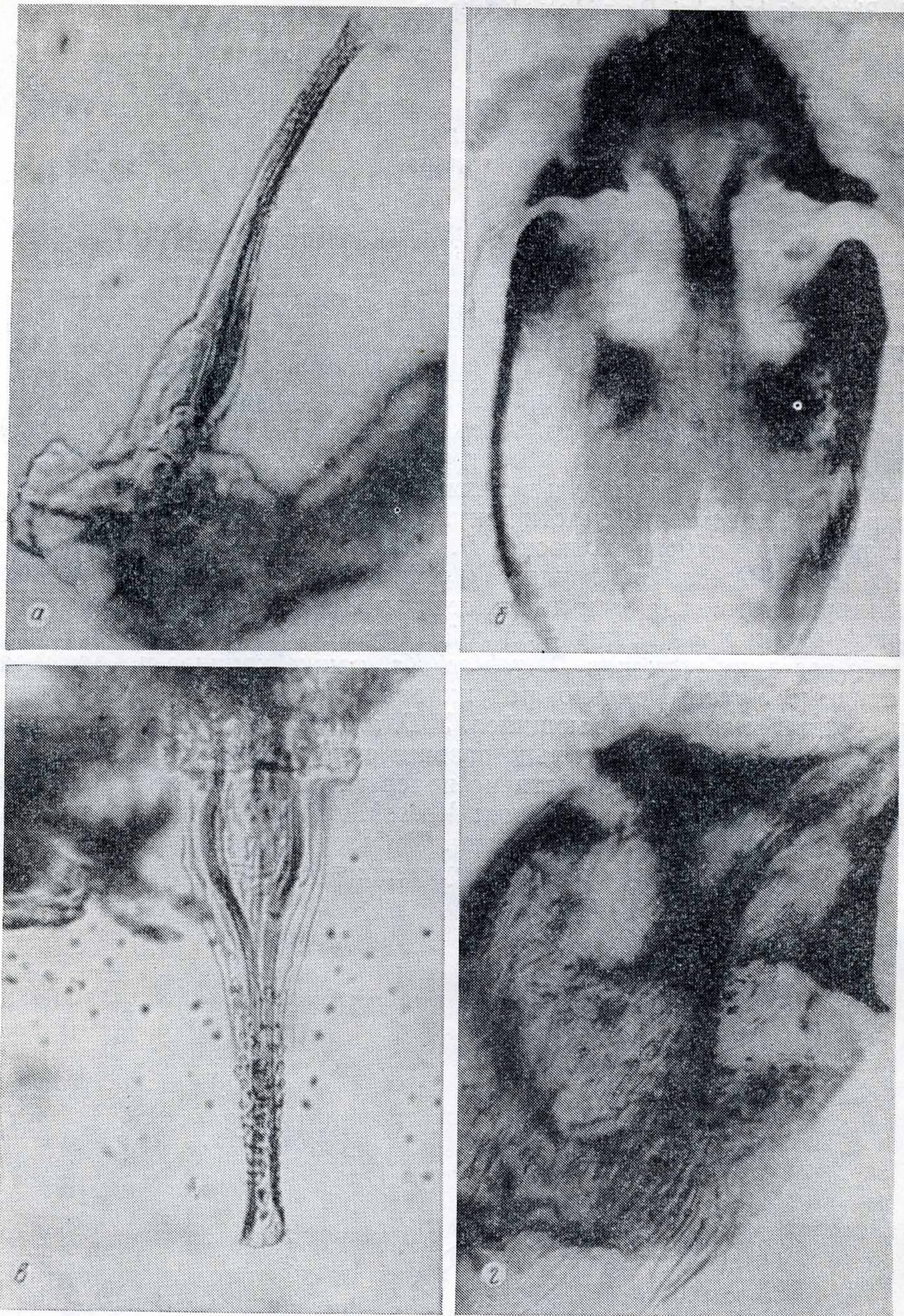
Рис. 5. Детали строения терминалий самцов и самок Phytoecia badenкои Danilevsky, sp. n. (а — хлыст эндофаллюса; б — генитальный сегмент самки) и Ph. molybdaena (в, з — то же).
