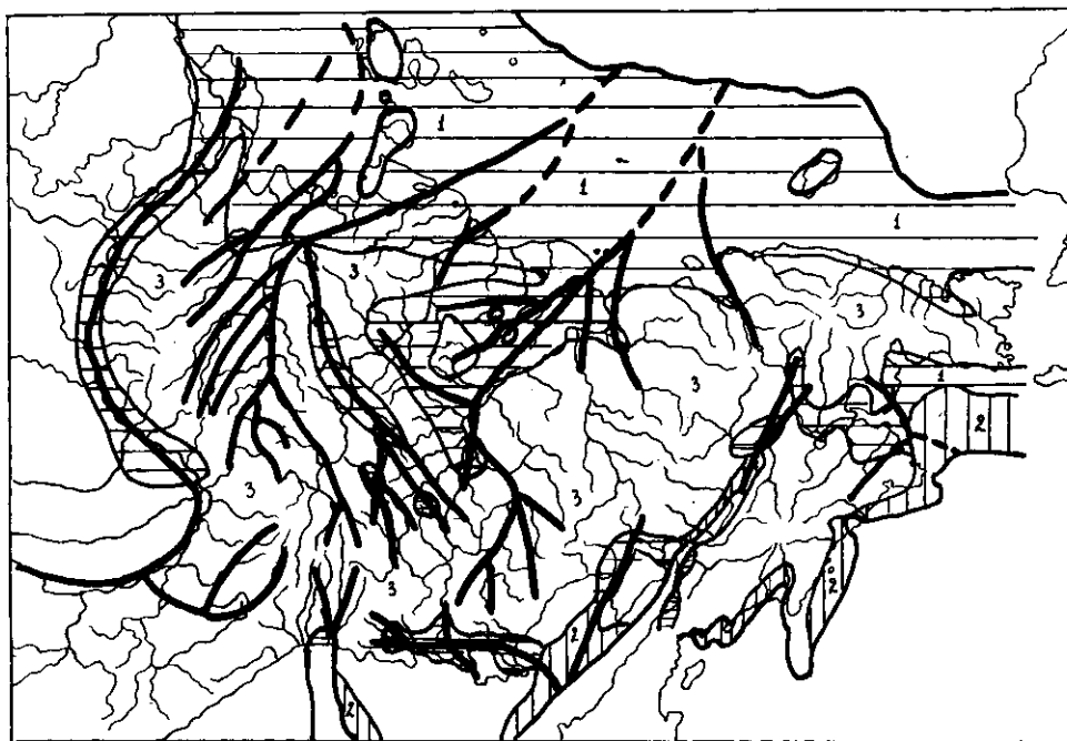
Рис. 8. Схема прости́рания речных долин в олигоцен-раннемиоценовом времени (из Барановой, Бискэ, 1964). 1 — озерно-речные равнины; 2 — прибрежные лагунодельтовые равнины; 3 — средние и низковысокие горы.
