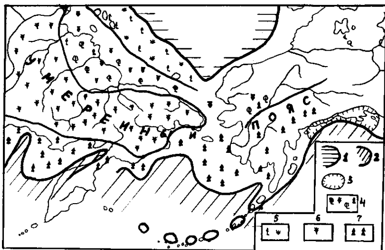
Рис. 4. Палеогеографическая схема Берингии для среднего и раннего плиоцена (из Барановой, Бискэ, 1964).
