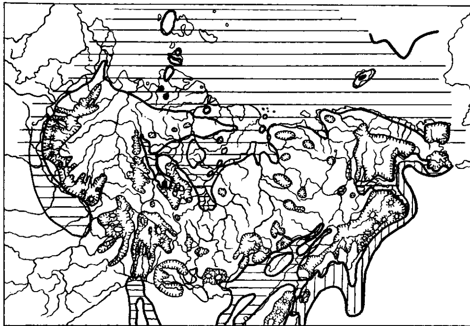
Рис. 11. Век среднечетвертичного (максимального) оледенения (из Барановой, Бискэ, 1964). Условные обозначения те же, что и на рис. 8.
