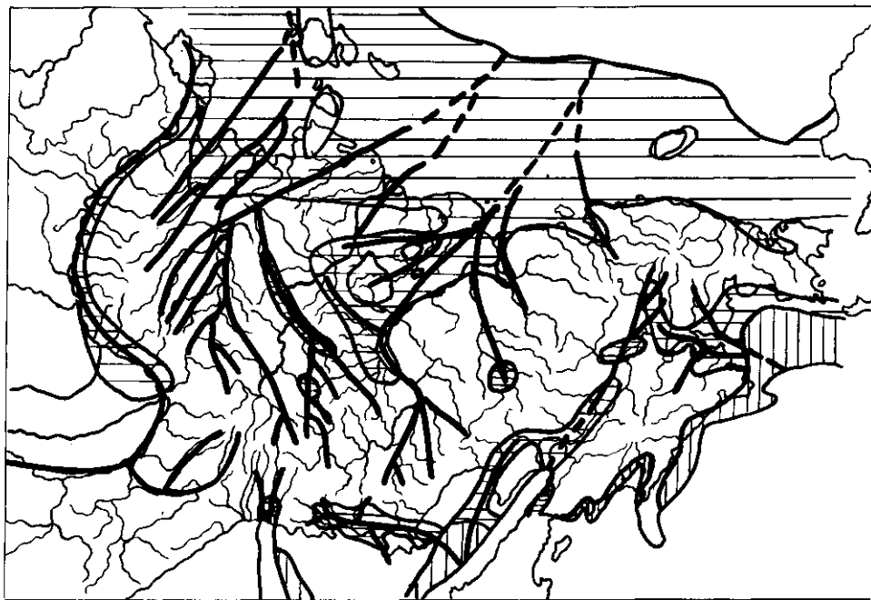
Рис. 9. Схема простираия речных долин первой половины плиоценовой эпохи (из Барановой, Бискэ, 1964). Условные обозначения те же, что и на рис. 8.
