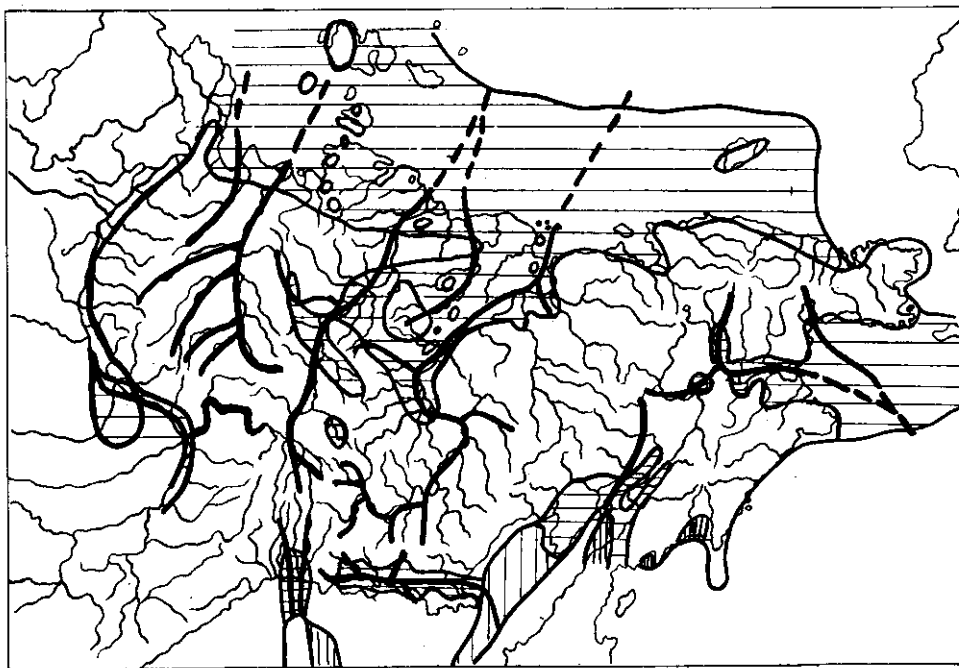
Рис. 10. Схема простираия речных долин конца позднего плиоцена — начала раннечетвертичной эпохи (из Барановой, Бискэ, 1964).
