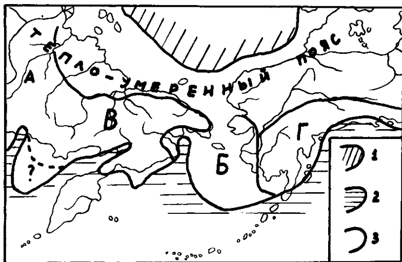
Рис. 2. Палеогеографическая схема Берингии для раннего-среднего миоцена (из Барановой, Бискэ, 1964).
