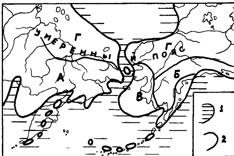
Рис. 3. Палеогеографическая схема Берингии для позднего миоцена (из Барановой, Бискэ, 1964).
