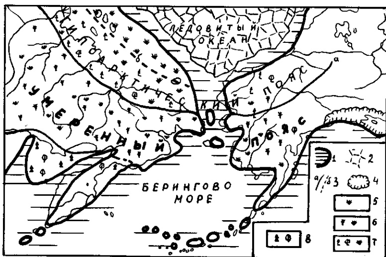
Рис. 5. Палеогеографическая схема Берингии для конца позднего плиоцена (из Барановой, Бискэ, 1964).
