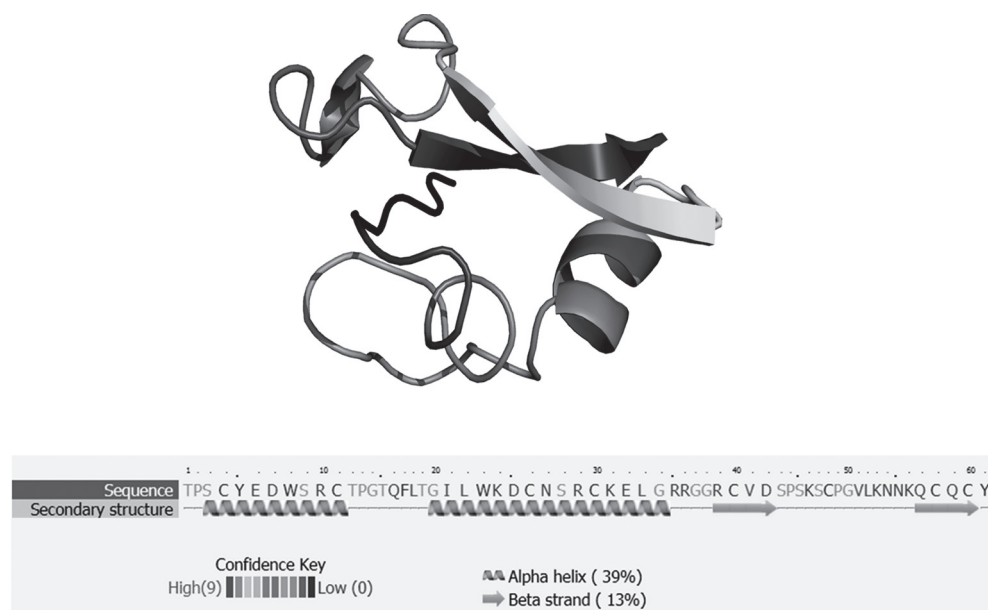
Рисунок 5. Трехмерная модель гирудомацина пиявки Hirudo nipponica , предсказанная с помощью Phyre2 (Kelley et al., 2015) на основе аминокислотной последовательности, транскрипированной из кДНК MH686152.
