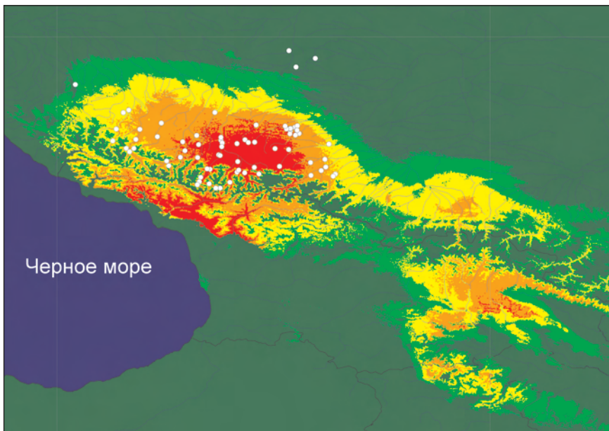
Рис. 1. Карта прогнозируемой области географического распространения Darevskia saxicola на Кавказе, построенная с применением программы Махент 3.3.3е. Области с красной (высокая), желтой (средняя) и светло-зеленой (низкая вероятность) заливкой – предполагаемая подходящая территория; белые точки – места находок
