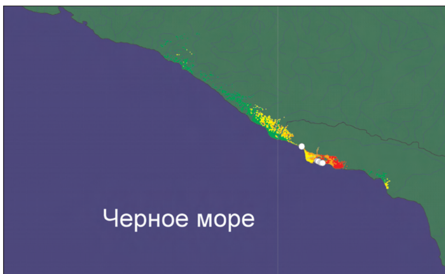
Рис. 6. Карта прогнозируемой области географического распространения Darevskia b. myusserica на Кавказе, построенная с применением программы Maxent 3.3.3e. Условные обозначения см. рис. 1
